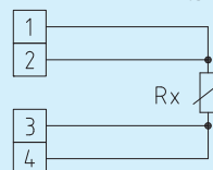
Схема подключения 1 четырехпроводное подключение (опционально)
