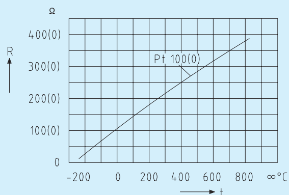
Характеристические кривые
