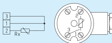
Схема подключения 1 трехпроводное подключение
