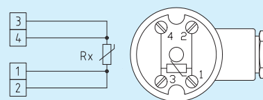
Схема подключения 1 четырехпроводное подключение
