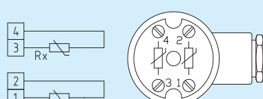
Схема подключения 2 двухпроводных подключения
