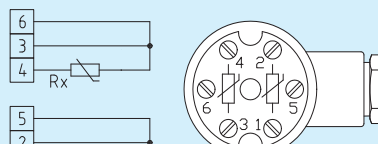
Схема подключения 2 трехпроводных подключения
