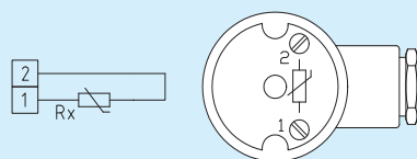
Схема подключения 1 двухпроводное подключение
