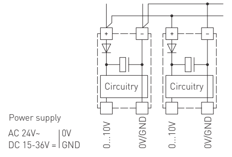
Схема соединения
